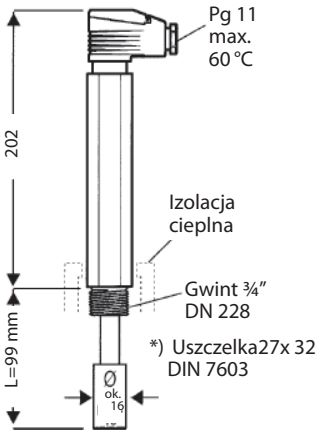
Elektroda pomiaru przewodności typ ERL 16-1, ¾"
