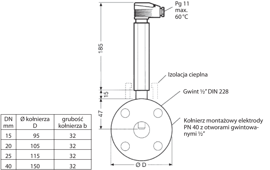
Elektroda pomiaru przewodności typ ERL 16-1 z kołnierzem montażowym, PN 40, DIN 2527
