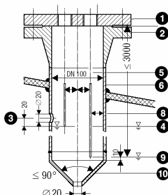
Rys. 5 Rura osłonowa elektrody zastosowanej jako ogranicznik poziomu w połączeniu z elektrodą regulacją poziomu lub alarmu wysokiego poziomu
